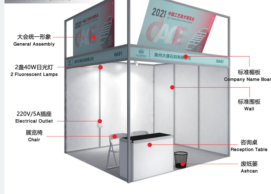
标准展位 (3mX3m) 解析图 Standard Booth (3mX3m)
